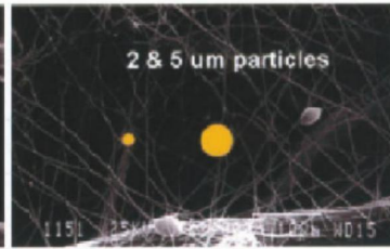
Высокая первоначальная фильтрация, по ГОСТу 5011 эффективность фильтрации доходит до 99,99%
