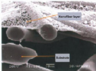
Нанометрический материал фильтра Kerry при увеличении в 1100 раз
